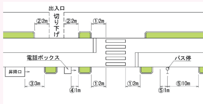
図Ⅲ-2 植樹帯設置を避けるべき範囲
